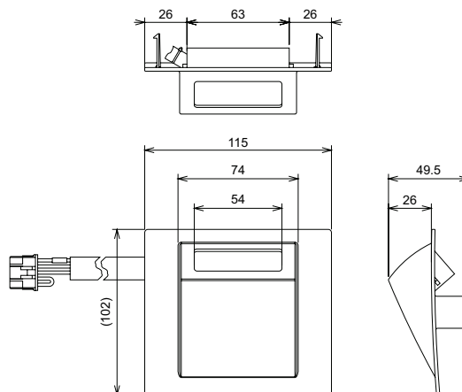
Kit Sensor de Presença SOR-NEP
