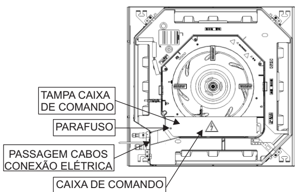
VISTA POR BAIXO SEM O PAINEL DE AR
